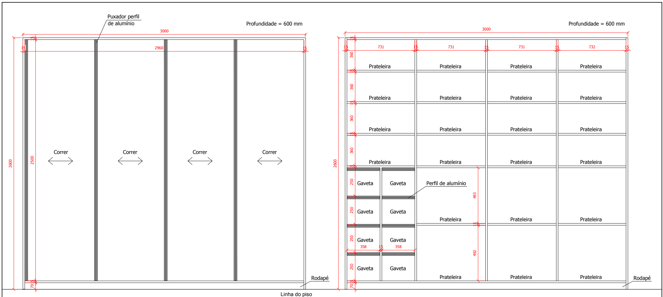
Vista Frontal - Armário 01 SEM ESCALA
